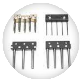
PINNHÅLLARE
